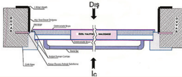
İçten Pervazlı Yangın Kapısı Kesit Resmi Internal Fire Door Section
