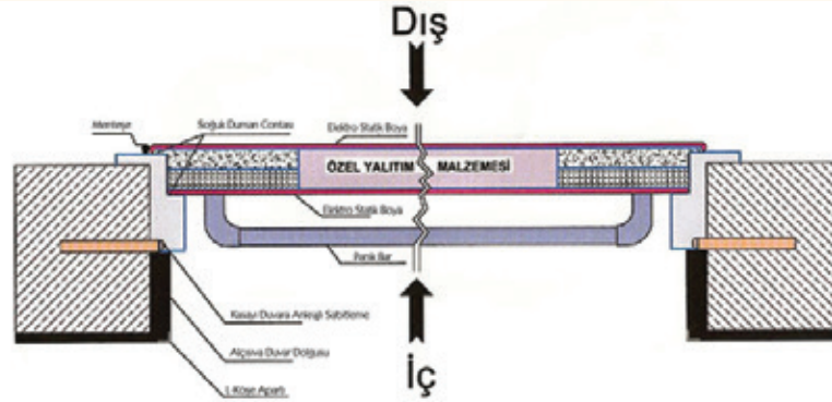
İçten Pervazlı Yangın Kapısı Kesit Resmi Internal Fire Door Section
